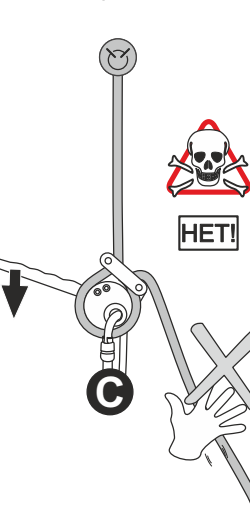
Рис. 13. Блокировка устройства
