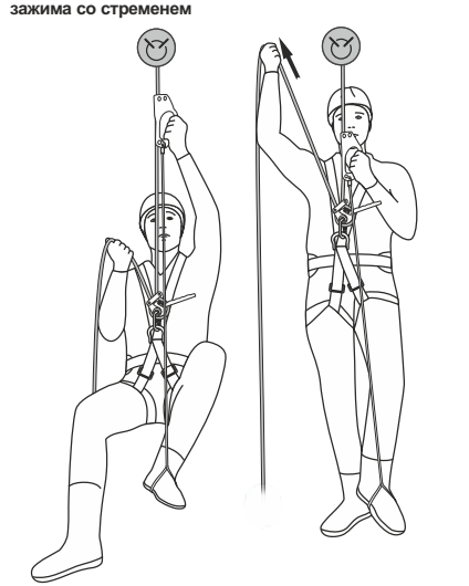
Рис. 11. Подъем с использованием зажима со стремнем
