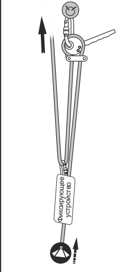
Рис. 12. Простой полиспаст
